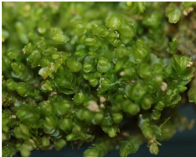
Nardia scalaris
